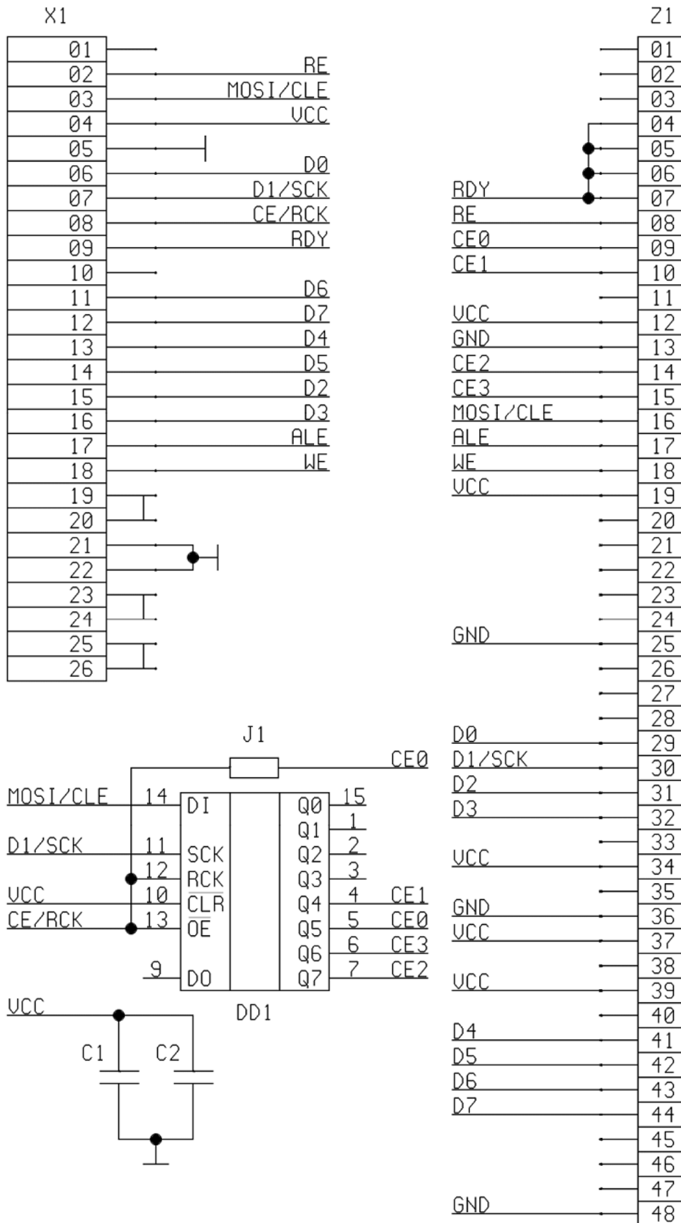
Схема электрическая принципиальная
